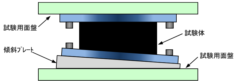
図-2 免震部材の傾斜実験概要
