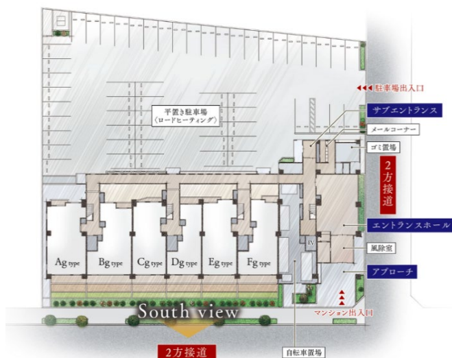
敷地配置図
