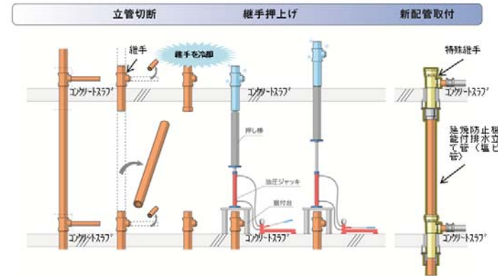
「HK-D工法」の作業手順
