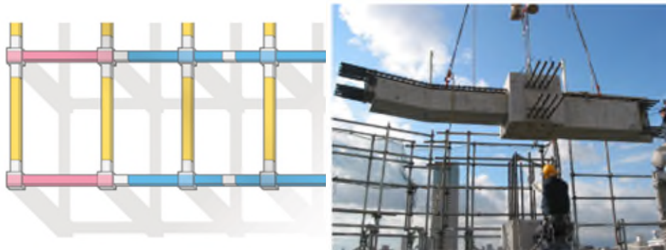
PCa梁の分割イメージ（青、赤、黄に分割）
